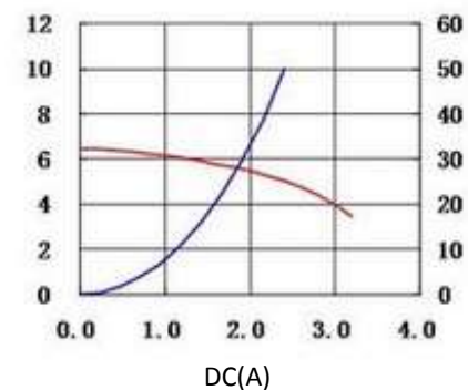
8. CD6020MBDS-220MC
